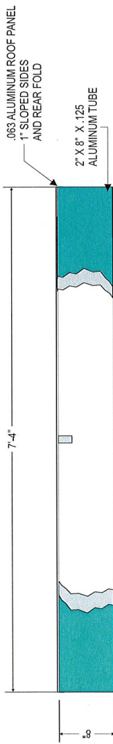
N4.a FRONT VIEW SCALE: 1"=1'
